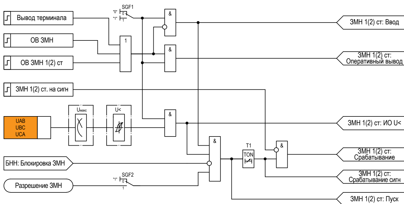
Рисунок 2.1 – Функциональная схема ступени ЗМН
