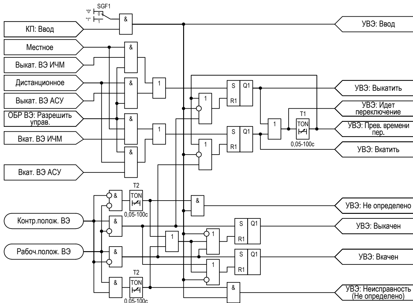
Рисунок 2.31 – Функциональная схема логики УВЭ
