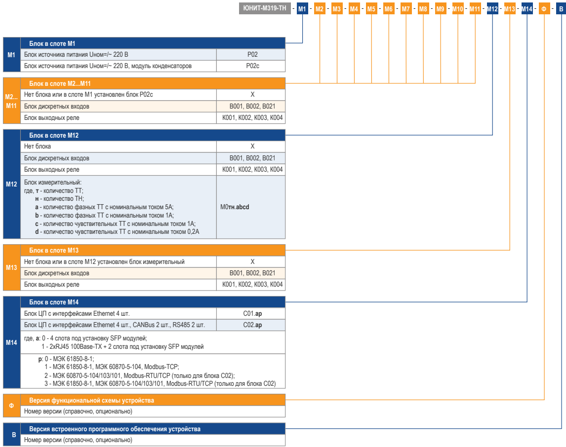
Рисунок Б.2 – Код заказа устройства «ЮНИТ-М319-ТН»
