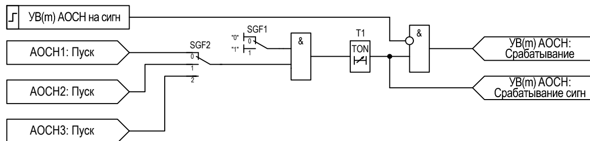
Рисунок 2.6 – Функциональная схема логики УВ АОСН
