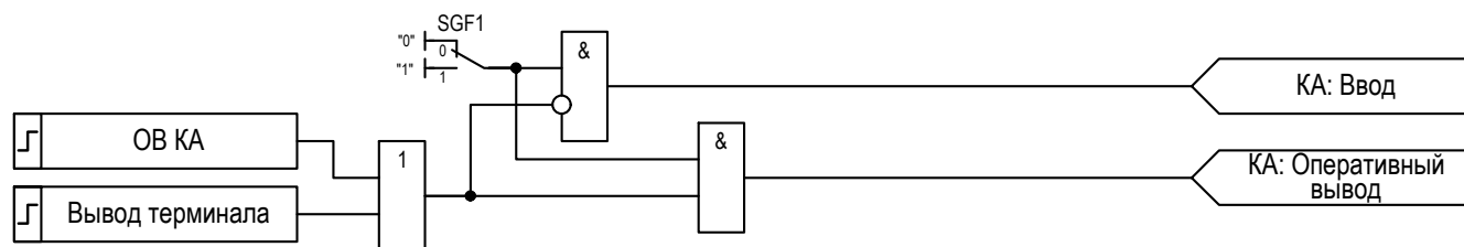
Рисунок 2.25 – Логика управления режимами КА
