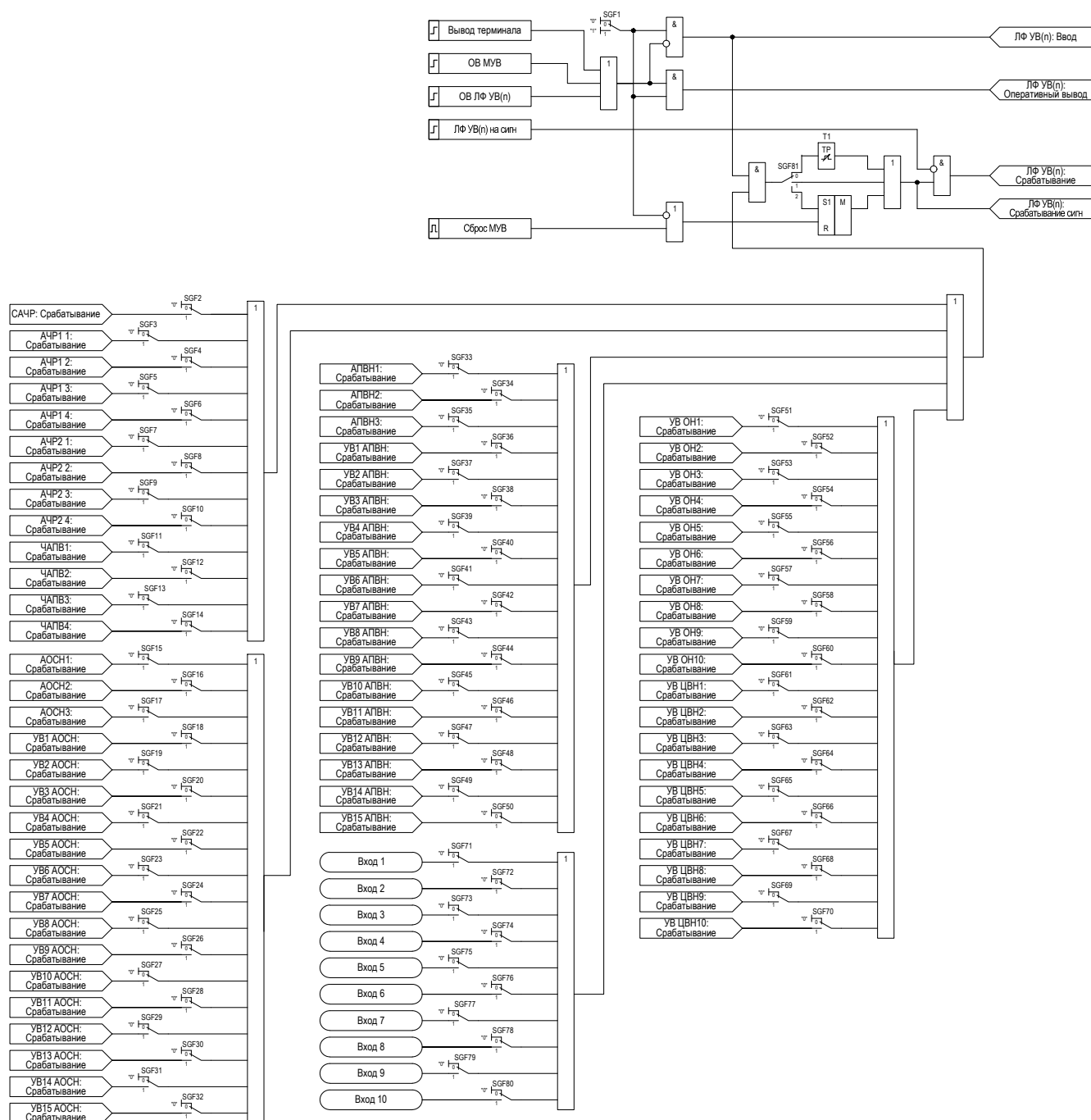
Рисунок 2.21 – Функциональная схема ЛФ УВ
